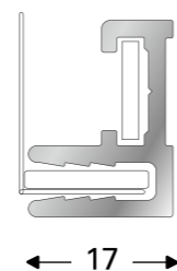
Intex 17 / 1-seitig, Oberfläche eloxiert
