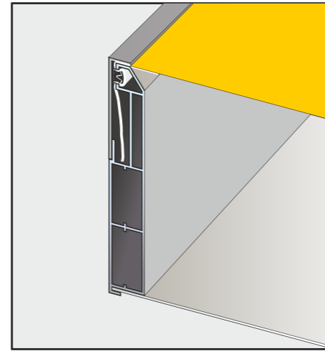
Schnittzeichnung Profil
