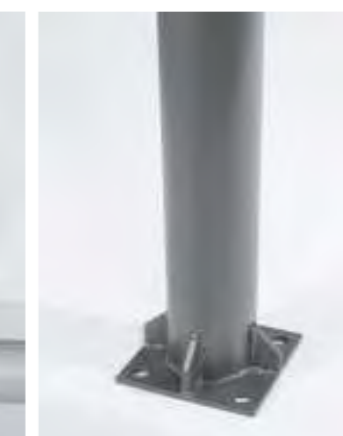
Sockelplatte mit Knoten- blechen und 16 mm Bohrungen.
